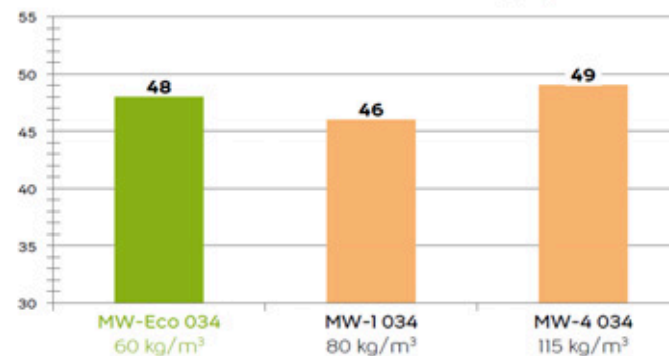
Schallmessungen EMPA Luftschalldämmung R_w + C_{tr} [dB]
