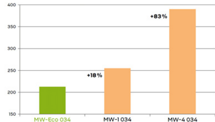
Grauenergiegehalt bei 200 mm Dämmung [MJ/m 2 ]
